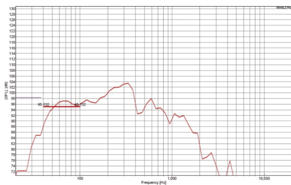
轴向频率响应
