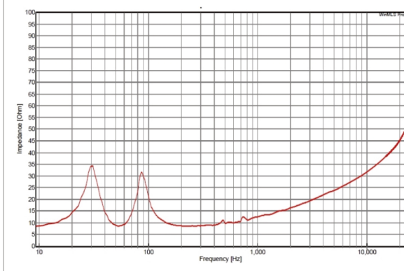
阻抗特性
